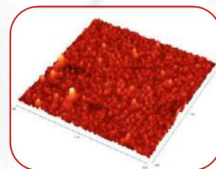
Nanolignin
