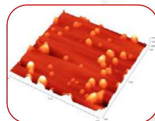
Nanocellulose
